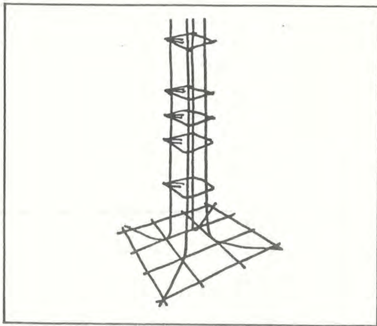
Anclaje de columnetas en zapata
