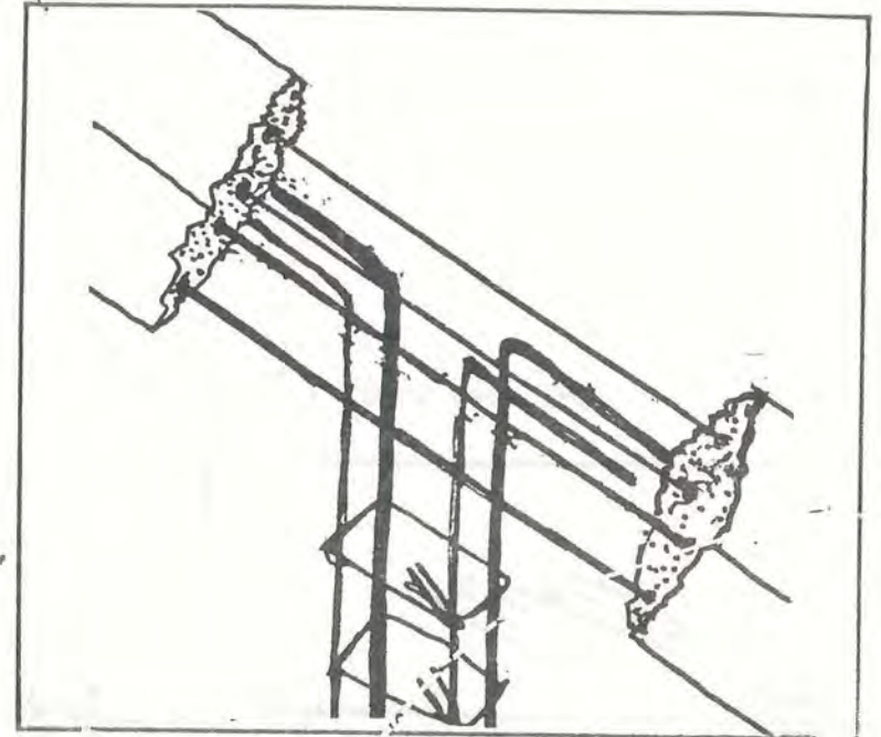
Anclaje de columneta nueva en viga existente
