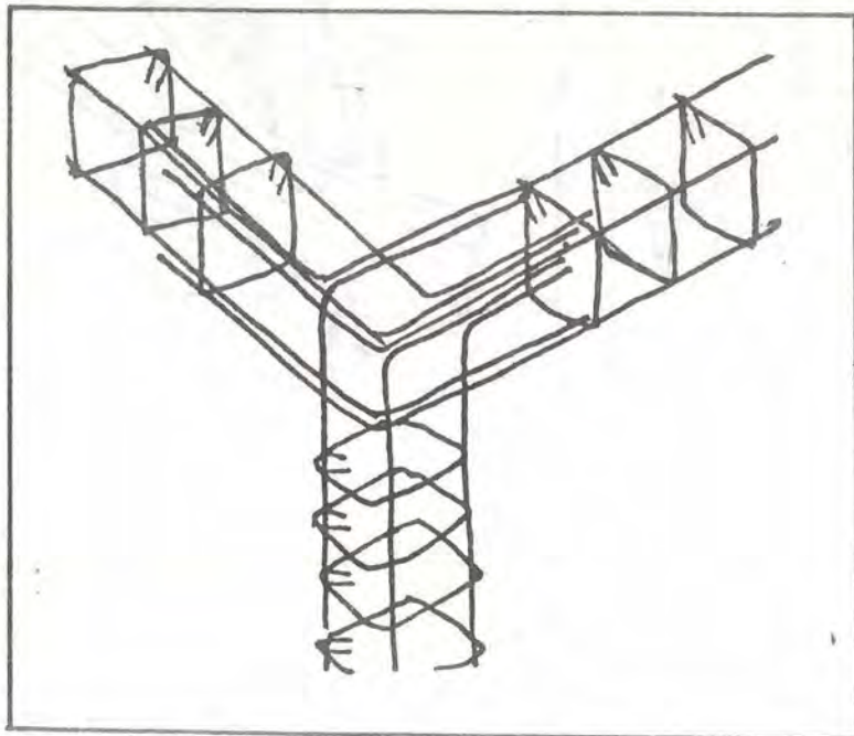
Unión de columneta con vigas de amarre en esquina
