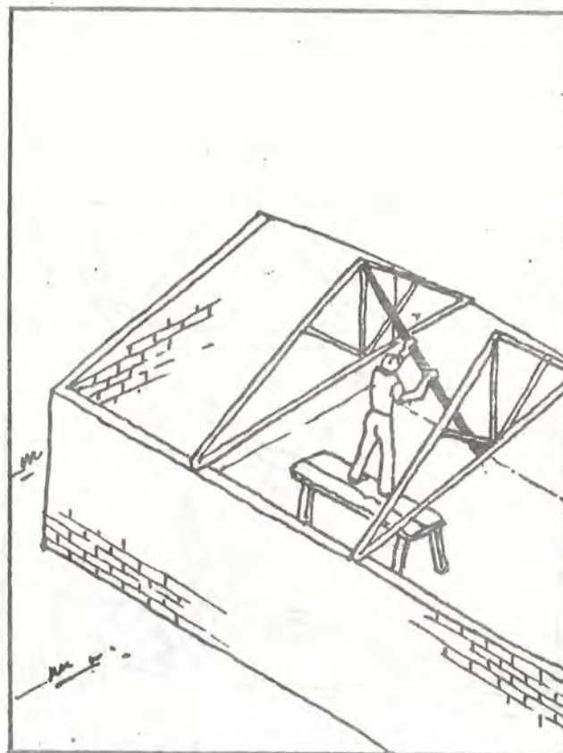
Coloque riostra (diagonal) entre cerchas
