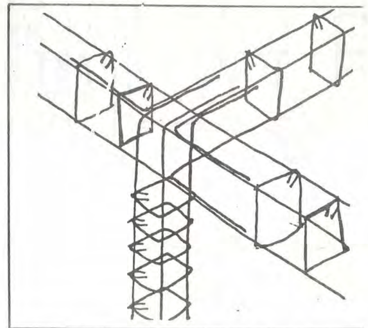
Unión de columneta con vigas de amarre en "T"
