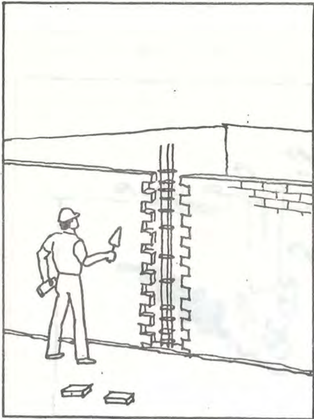
Verifique colocación correcta del castillo
