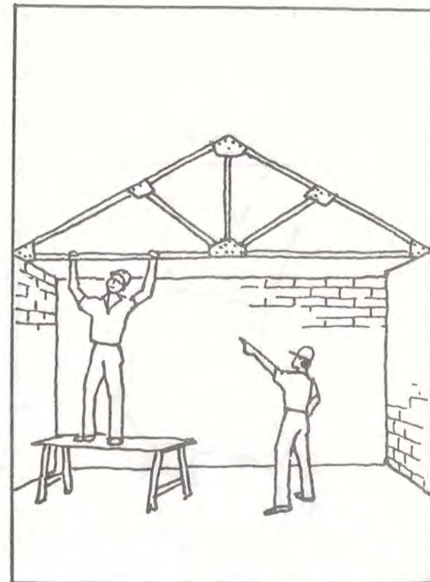
Coloque Cercha
